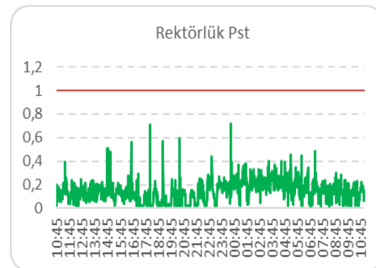
Şekil-19. Rektörlük Pst
