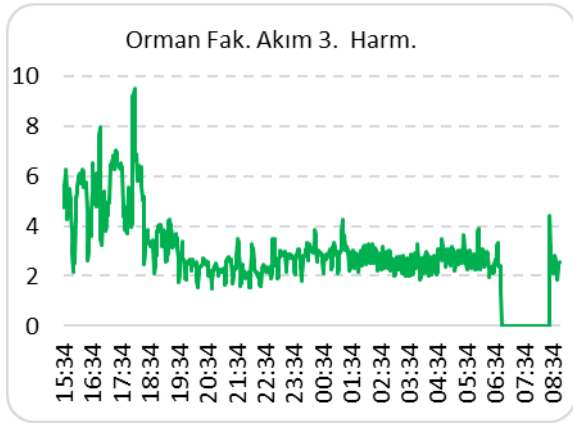
Şekil-10. Orman Fak. 3. Harmonik
